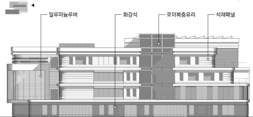
우측면도 SCALE:1/500
