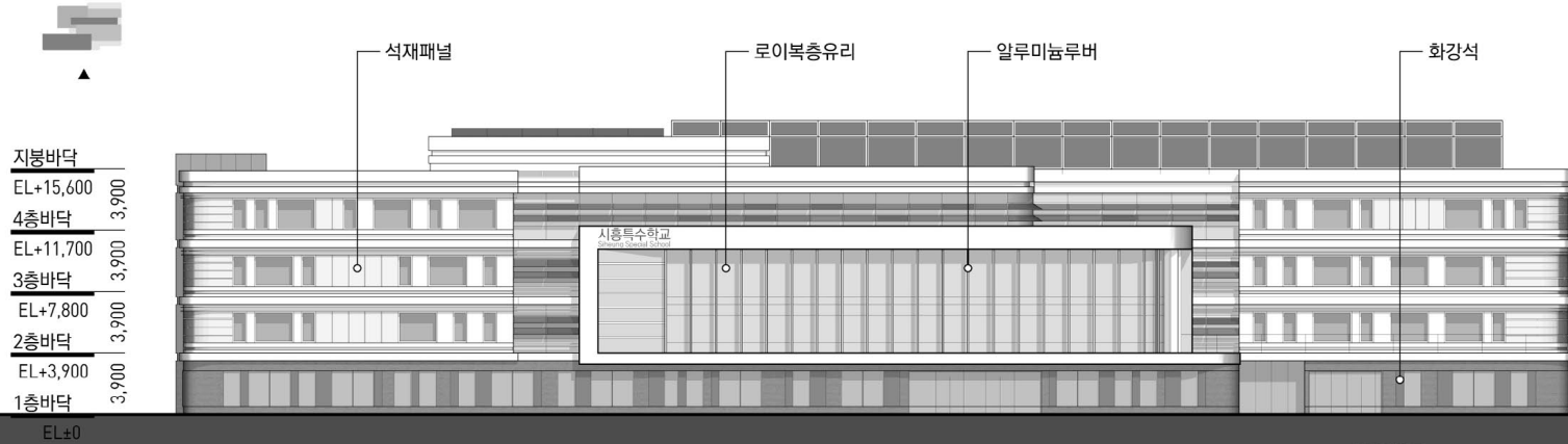
정면도 SCALE:1/500
